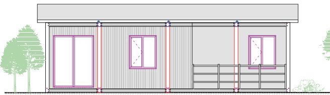
FRONTANSICHT
