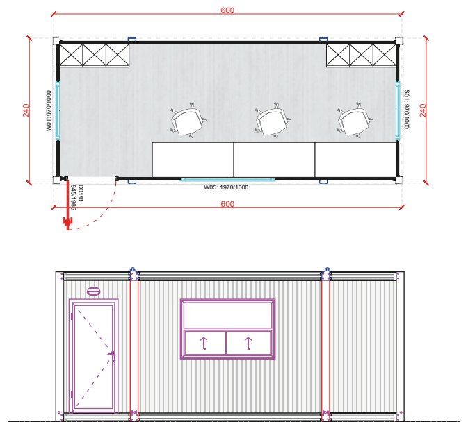
FRONTANSICHT
