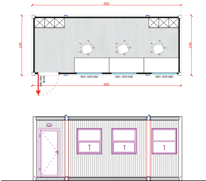
FRONTANSICHT
