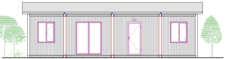
FRONTANSICHT
