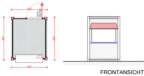
FRONTANSICHT
