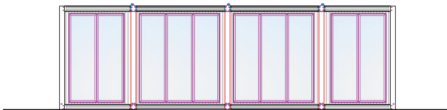
FRONTANSICHT
