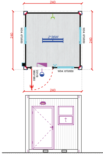
FRONTANSICHT
